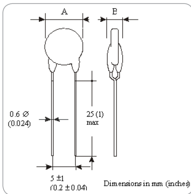
Type TQ Dimensions
