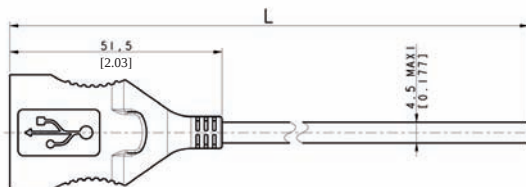
Part Number : USBAP 6 xxx Open
