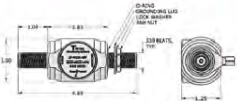
• LP-WBX-NFF 2000 - 6000MHz N Type F/F
